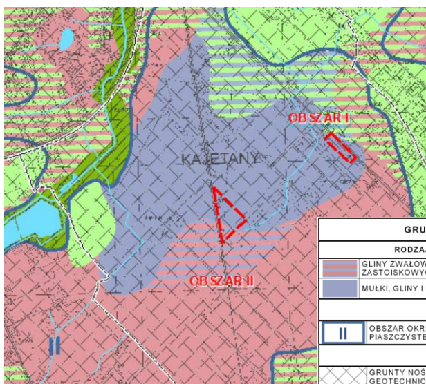
Rysunek 3 Warunki geologiczne
